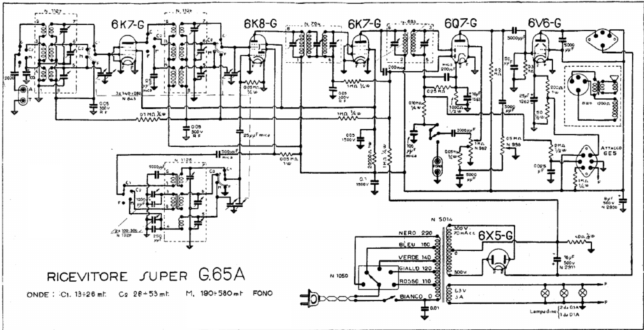
Lo schema elettrico.
